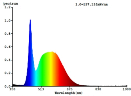
SPL62X62-48W-RGBWWW(at 6000k)
