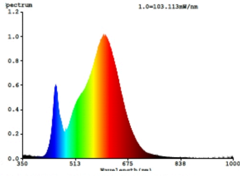
SPL62X62-48W-RGBWWW(at 3000k)
